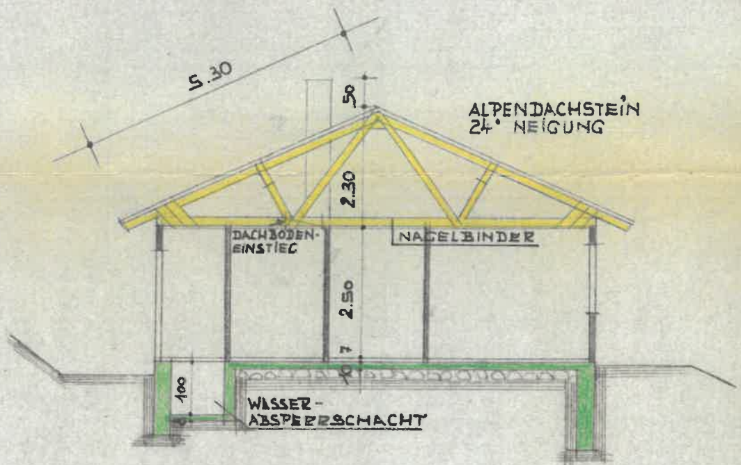
SCHNITT
